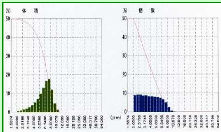
加工粉体粒度分布
