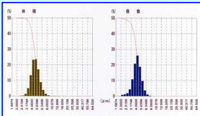
加工粉体粒度分布
